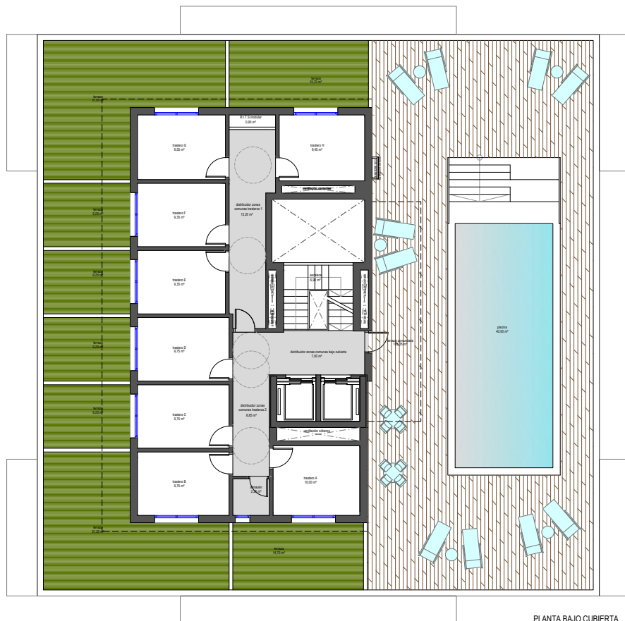
PLANTA BAJO CUBIERTA
