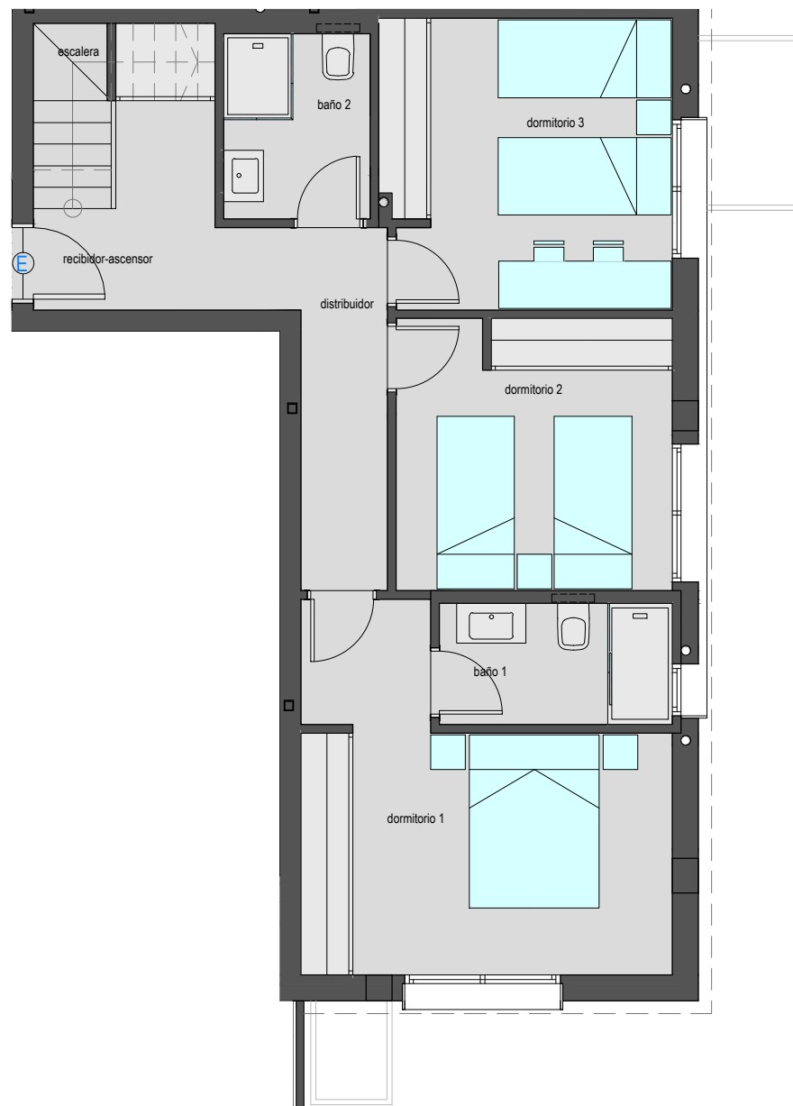
PLANTA 7ª
